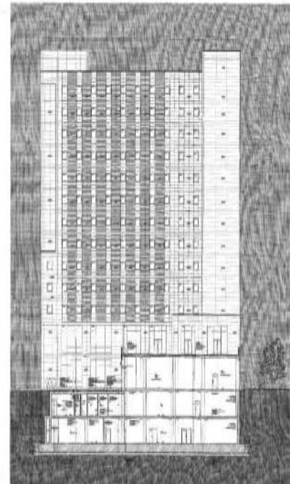
3-3 KESİTİ 1/100
